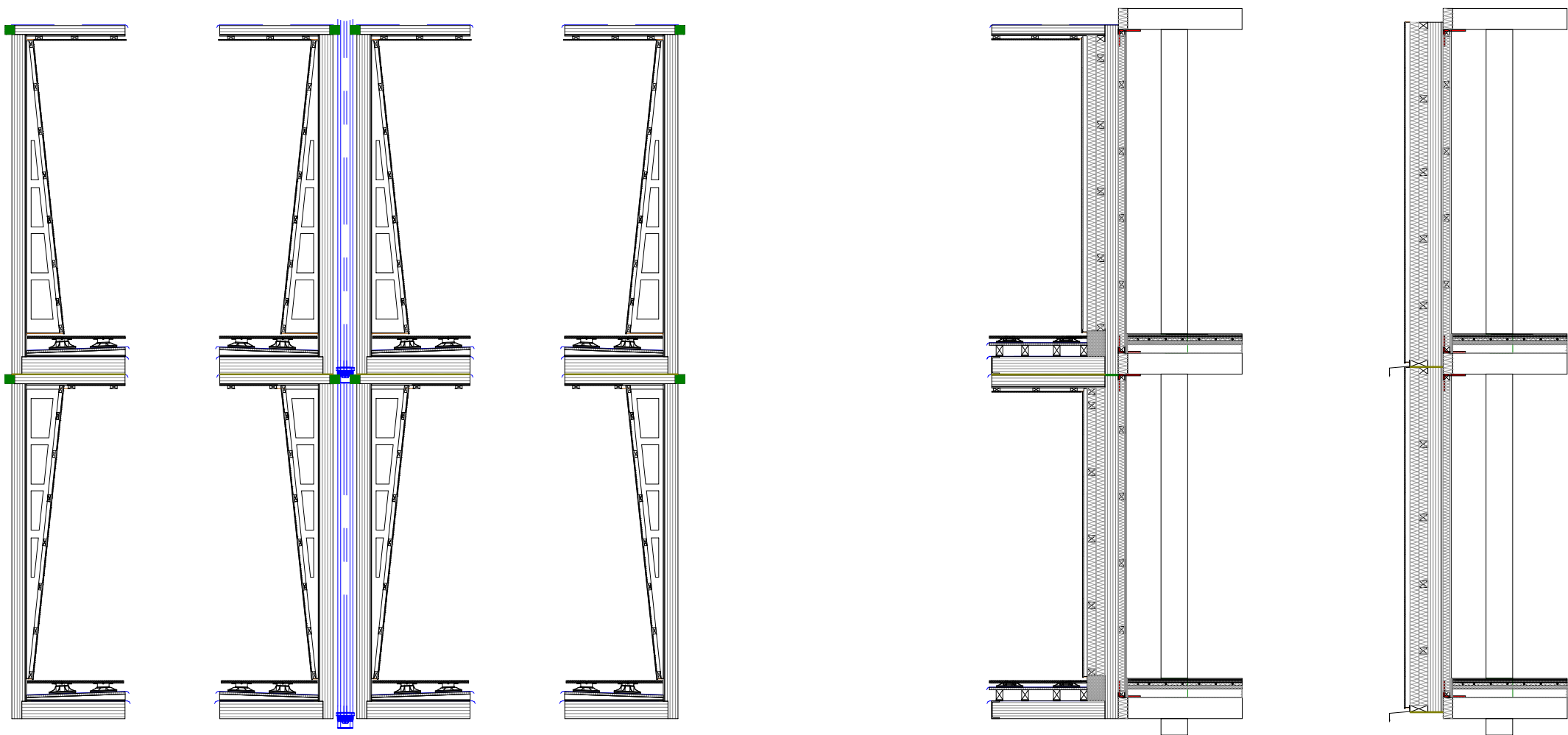
Lüftungsintegration
