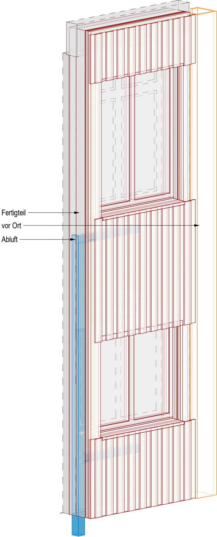
Paneltyp 3 mit Abluft
